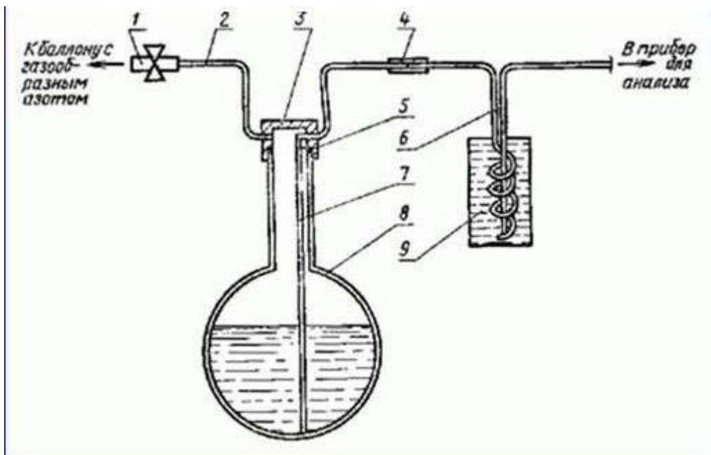
1 -трубка резиновая с зажимом; 2-медная трубка 6 × 1мм; 3 –крышка; 4 -трубка резиновая; 5-прокладка; 6 -испаритель; 7-трубка из нержавеющей стали 3 × 0,7 мм; 8-криогенный сосуд; 9 -сосуд с водой
