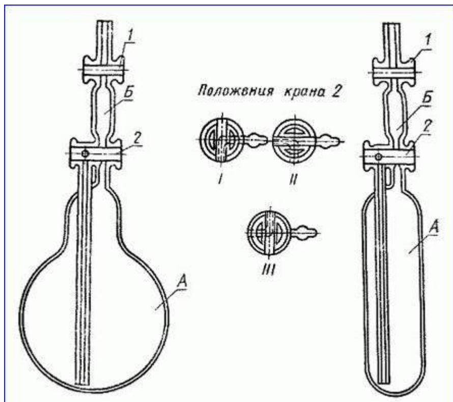
I -соединение сосуда A с атмосферой; II -кран закрыт; III -соединение сосуда A с сосудом B ; 1 -одноходовой кран; 2 -двухходовой кран.
