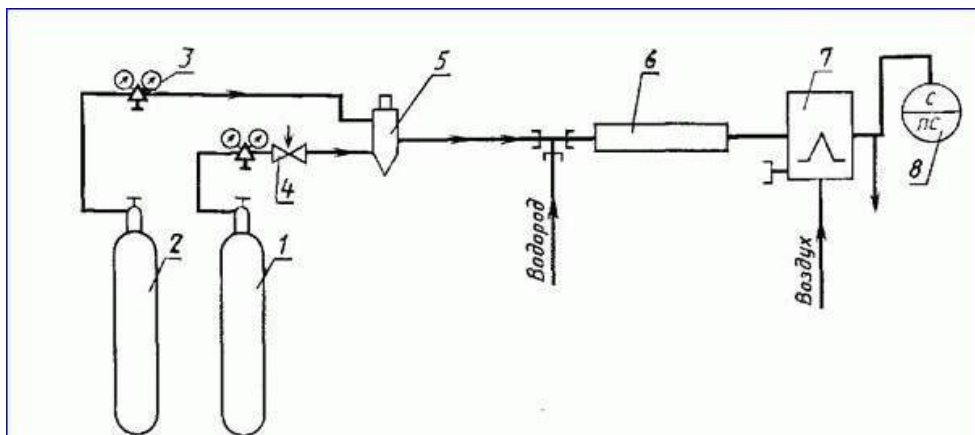
1 -баллон с анализируемый газом; 2-баллон с газом-носителем; 3-редуктор баллона; 4 - вентиль тонкой регулировки; 5-дозатор; 6-газохроматографическая колонка; 7-реактор; 8- детектор пламенно-ионизационный; 9 -измерительный прибор
